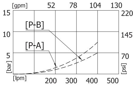
ΔP : 2012A
