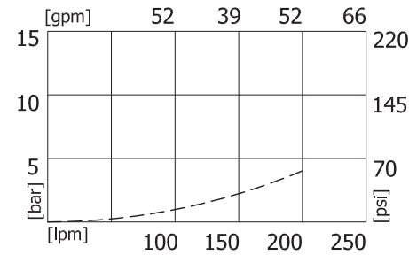
ΔP : 1212B
